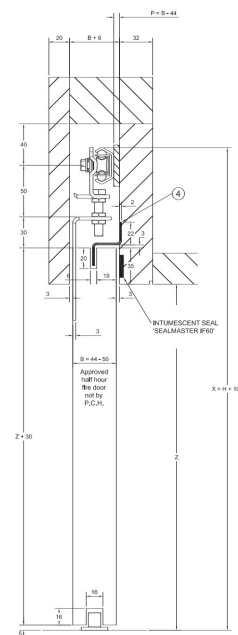
End Elevation
