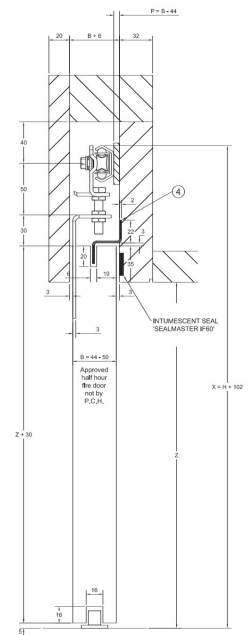
End Elevation
